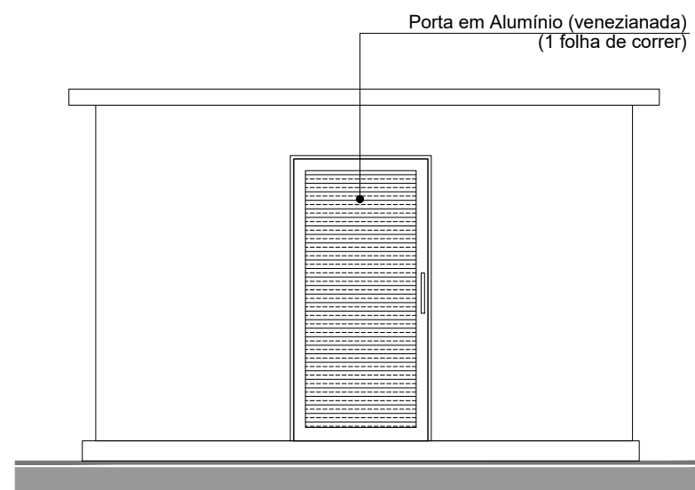
Abrigo ETE - Nereu Ramos Elevação Frontal escala 1:50
