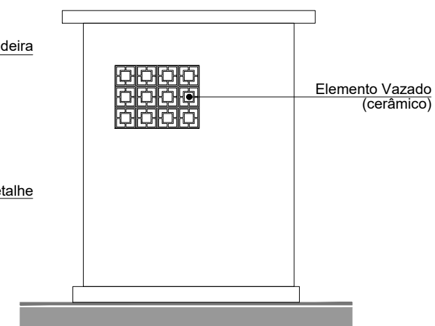
Abrigo ETE - Nereu Ramos Elevação Lateral (direita) escala 1:50
