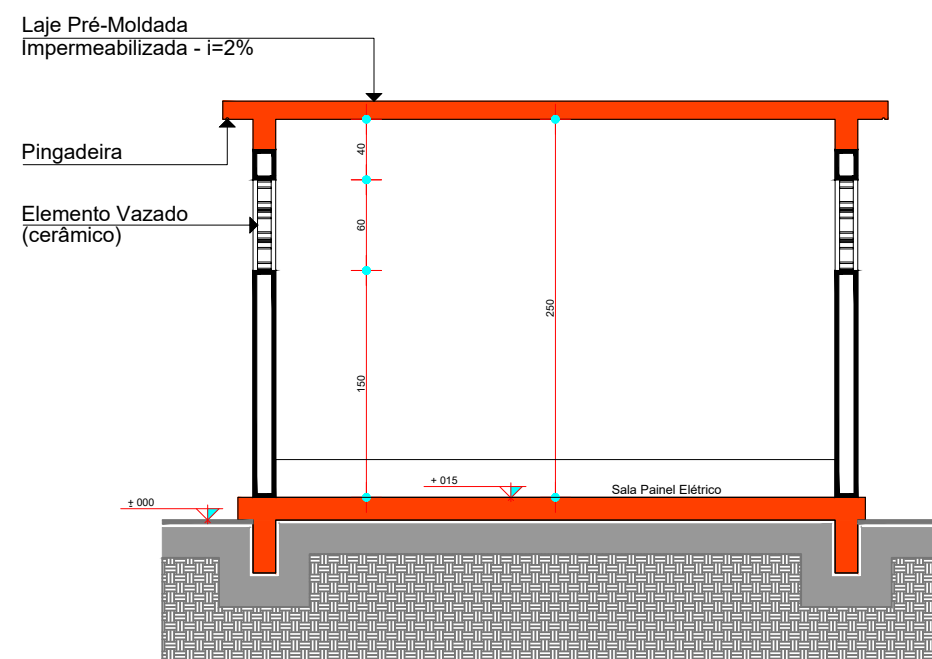
Abrigo ETE - Nereu Ramos Secção A escala 1:50
