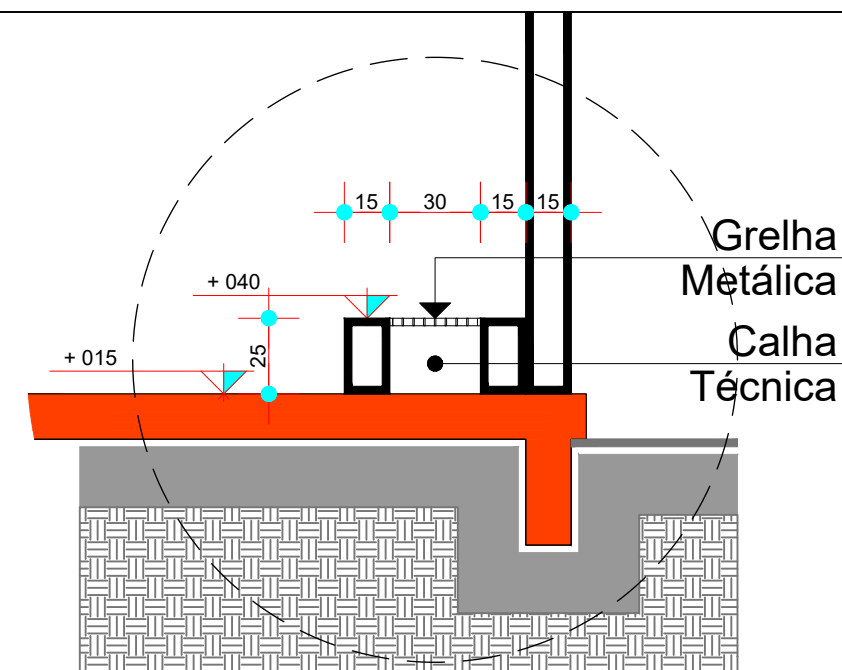
Detalhe Calha técnica escala 1:25
