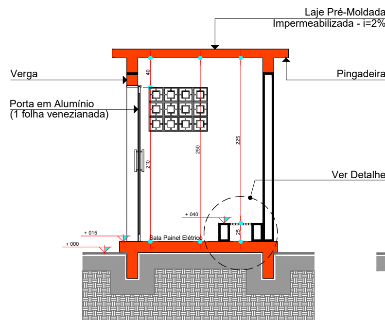
Abrigo ETE - Nereu Ramos Secção B escala 1:50
