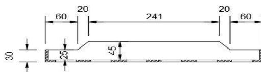
CORTE "AA"
