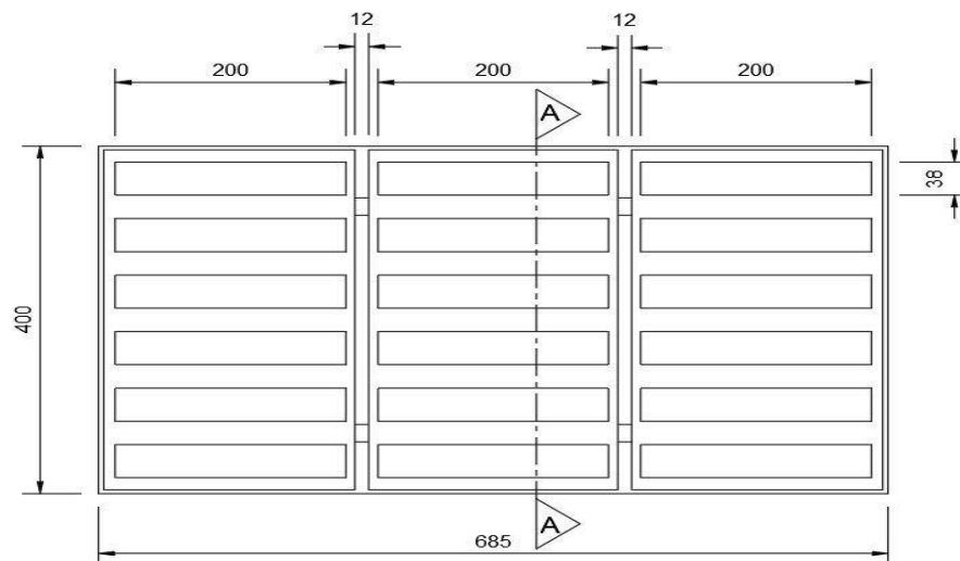
VISTA INFERIOR
