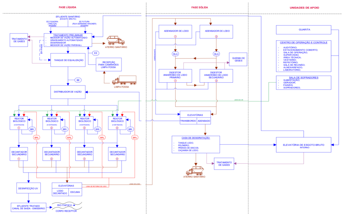
Imagem 06 – Fluxograma geral da estação.
