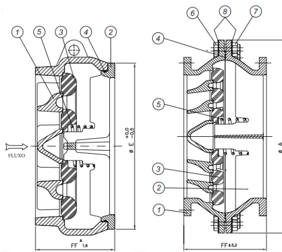
Figura 04 – Modelo de referência para válvula de retenção
