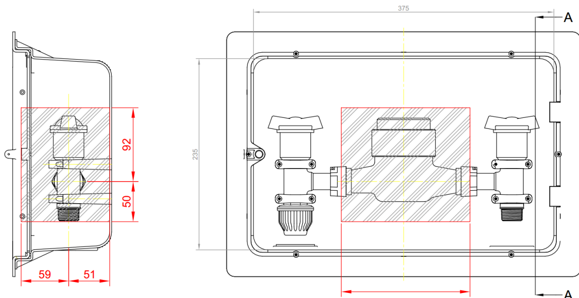
Figura 1 – Limites dimensionais do conjunto Filtro e Hidrômetros em relação ao eixo de conexão.
