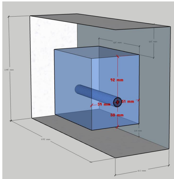
Figura 1 – Limites dimensionais do conjunto Filtro e Hidrômetros em relação ao eixo de conexão.
