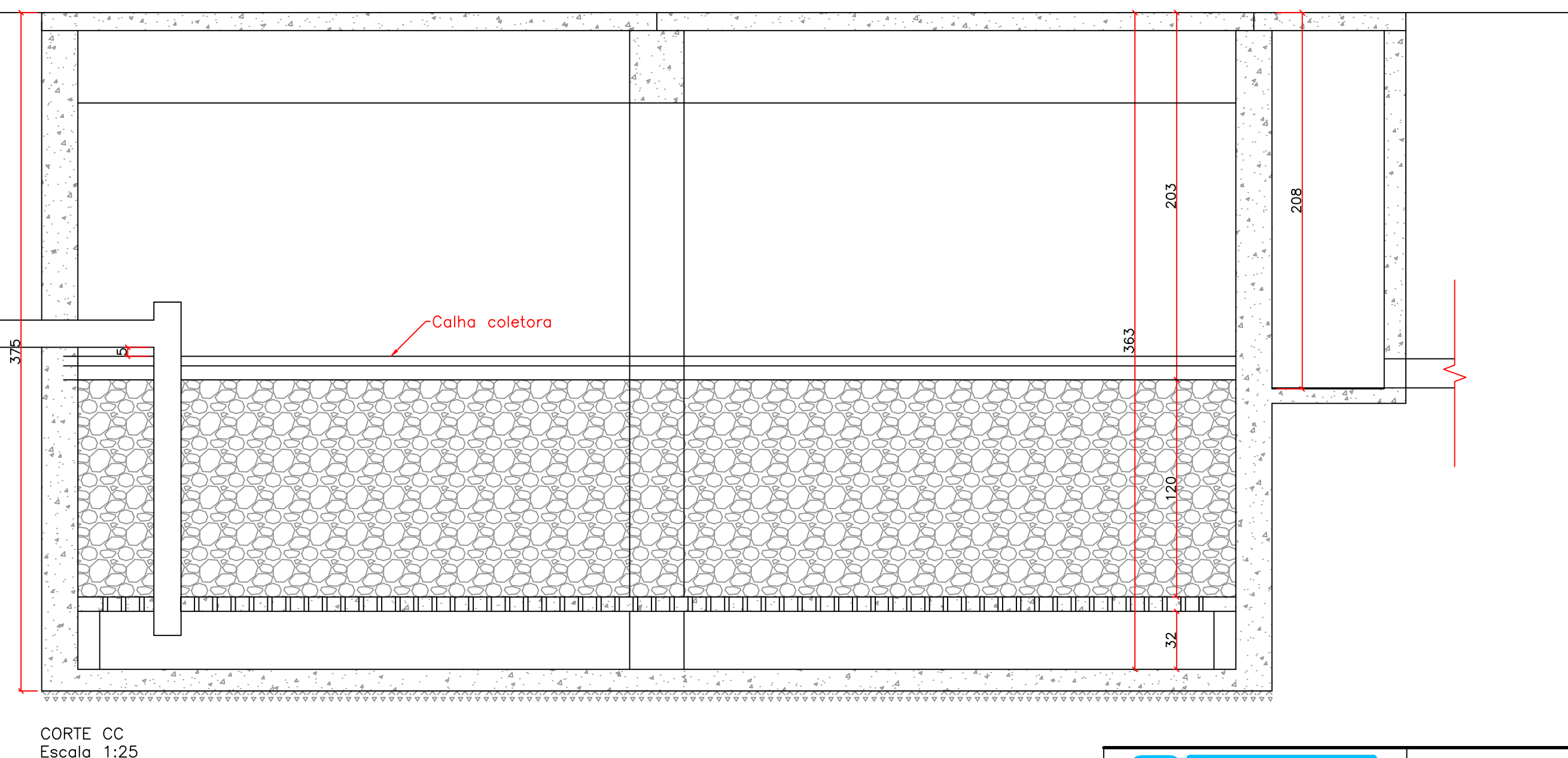
FILTRO ANAERÓBIO Escala 1:25
