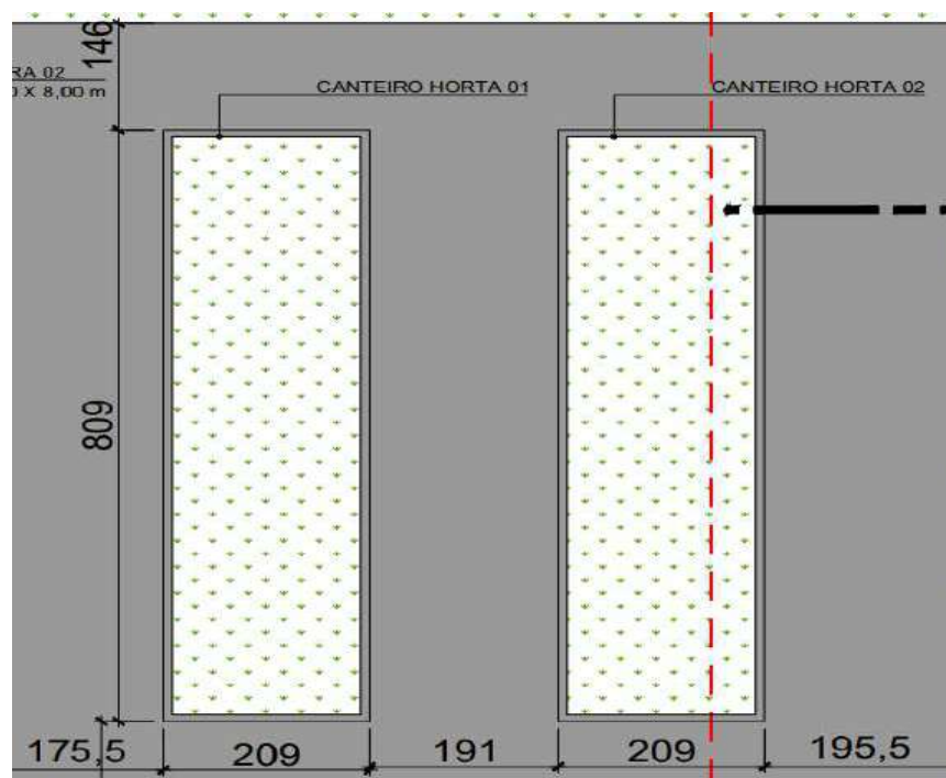
Figura 21 – Dimensões dos canteiros centrais da Horta Comunitária
