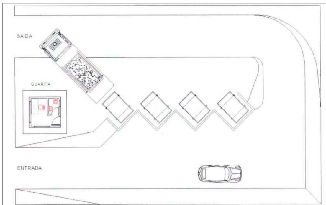
Figura 45 – Layout Básico de um PEV.
