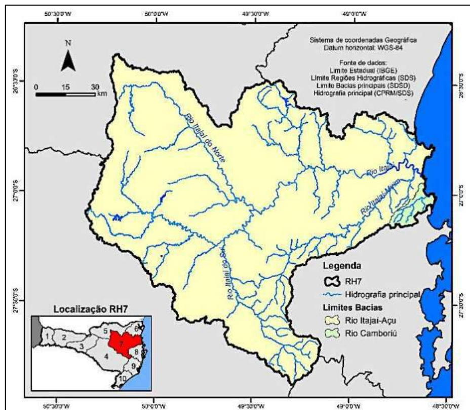
Figura 5 – Bacias hidrográfica de Rio do Sul/SC
