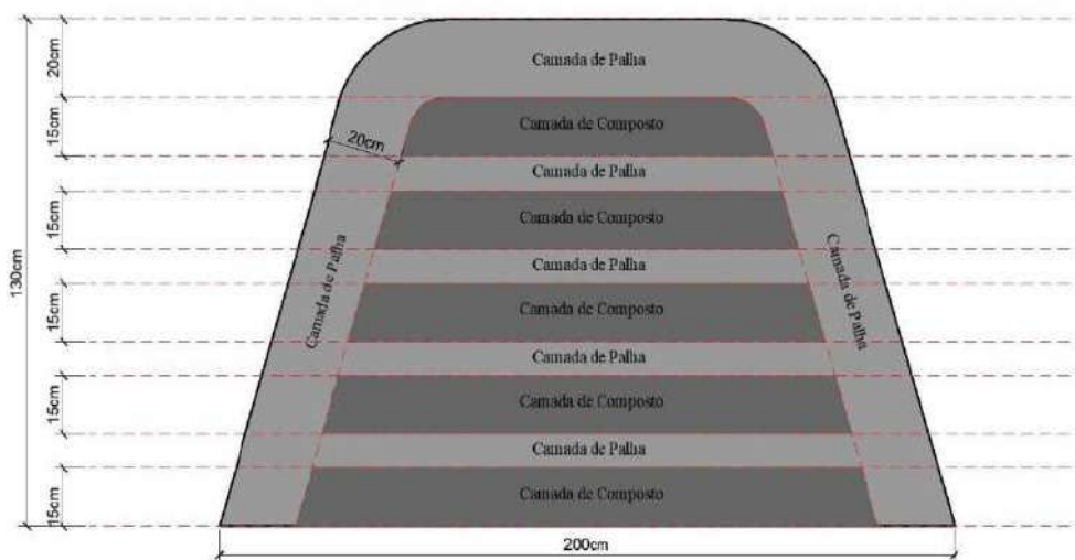
Figura 26 – Layout das camadas da leira de compostagem
