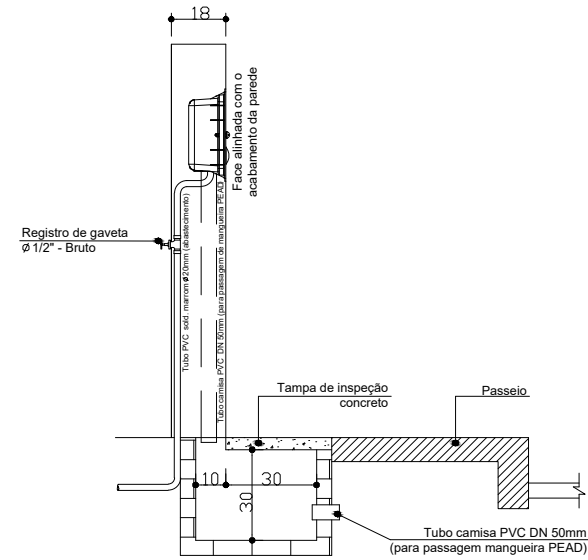
VISTA LATERAL ESCALA 1:25
