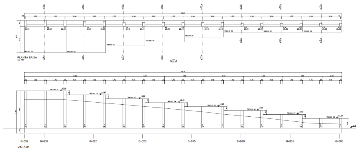
Imagem 05 – Planta baixa e vista frontal do muro de flexão a ser executado.
